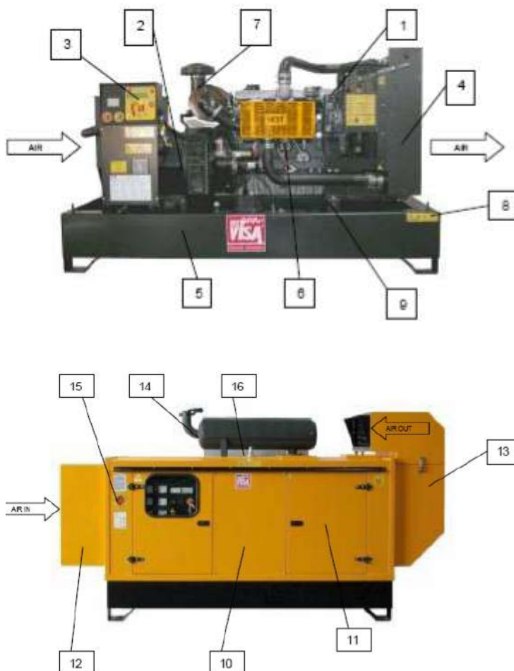
Рис.1 Основные части
