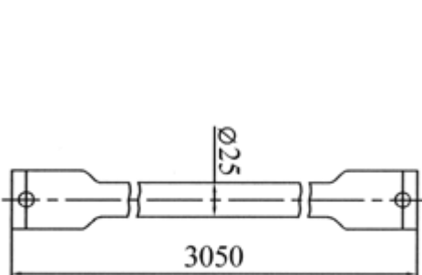
Связь горизонтальная
