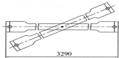
Связь диагональная
