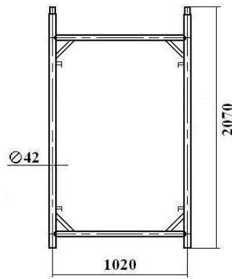
Рама проходная
