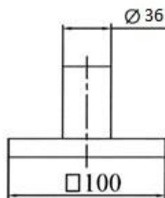
Рама проходная
